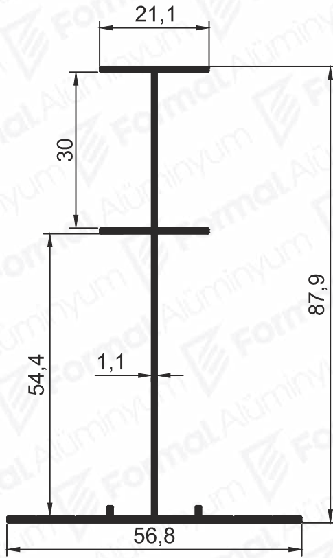
Pr.No: 2457 0,589 kg/m
