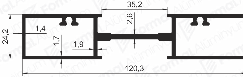
Pr.No: 2459 1,590 kg/m
