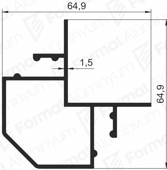
Pr.No: 8863 0,945 kg/m
