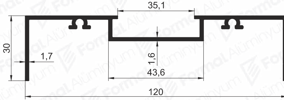
Pr.No: 2458 1,021 kg/m
