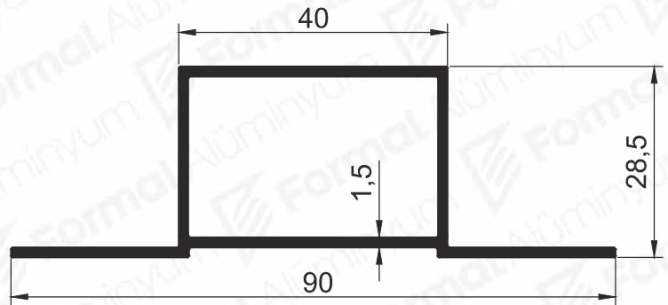
Pr.No: 9193 0,23 kg/m
