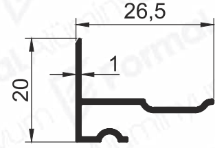
Pr.No: 8864 0,154 kg/m
