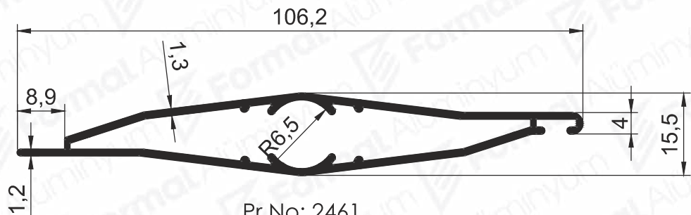
Pr.No: 2461 0,62 kg/m
