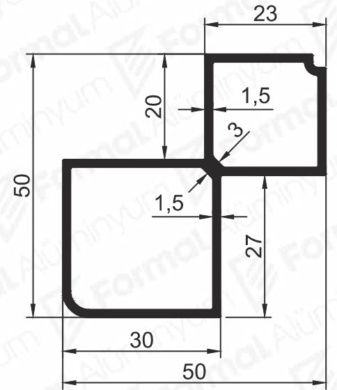
Pr.No: 2655 0,90 kg/m
