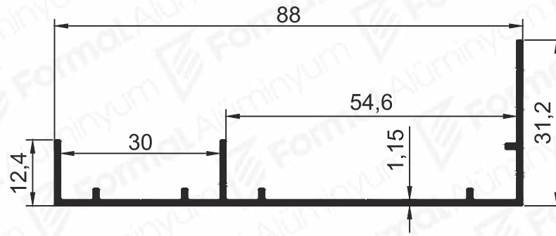
Pr.No: 2460 0,469 kg/m
