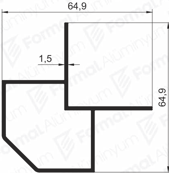
Pr.No: 9192 0,9 kg/m
